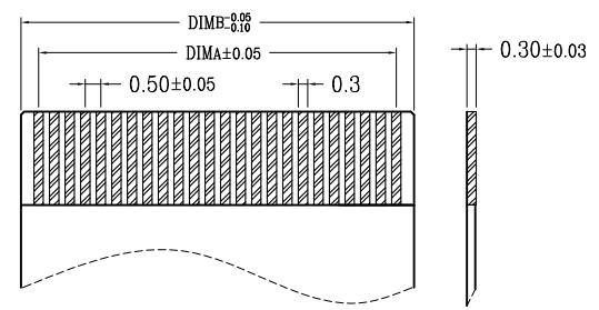
适用扁平线
